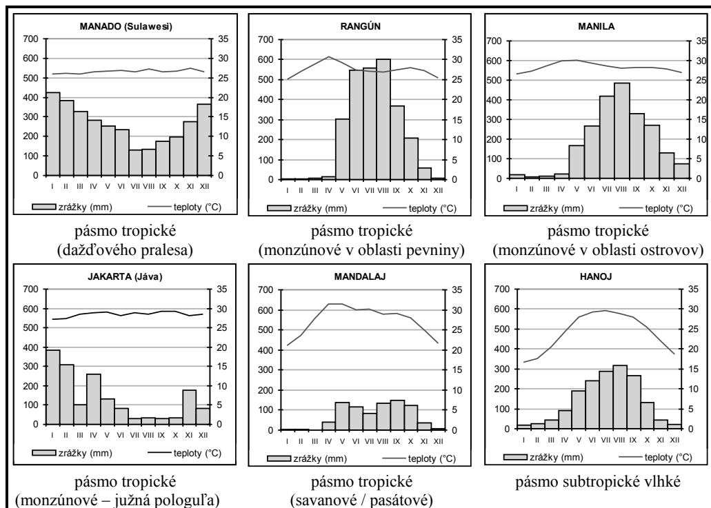
Obr. 39 Ročný chod teplôt a zrážok vo vybraných sídlach juhovýchodnej Ázie, Zdroj: World Weather 2014
