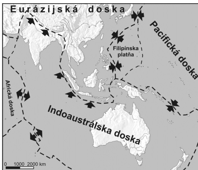
Obr. 38 Litosferické dosky v oblasti juhovýchodnej Ázie
