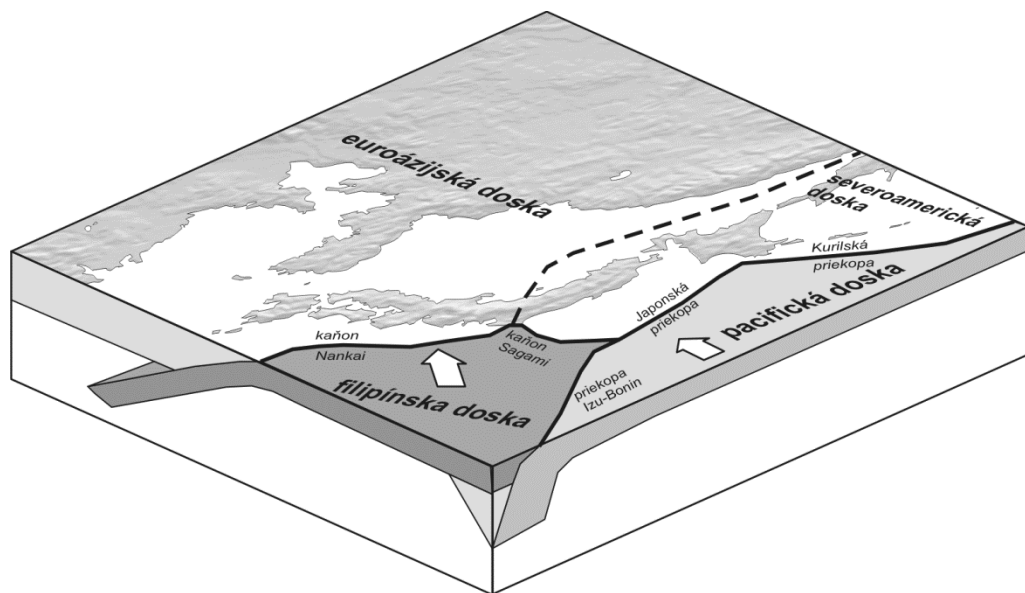
Obr. 66 Základná tektonická situácia Japonska
