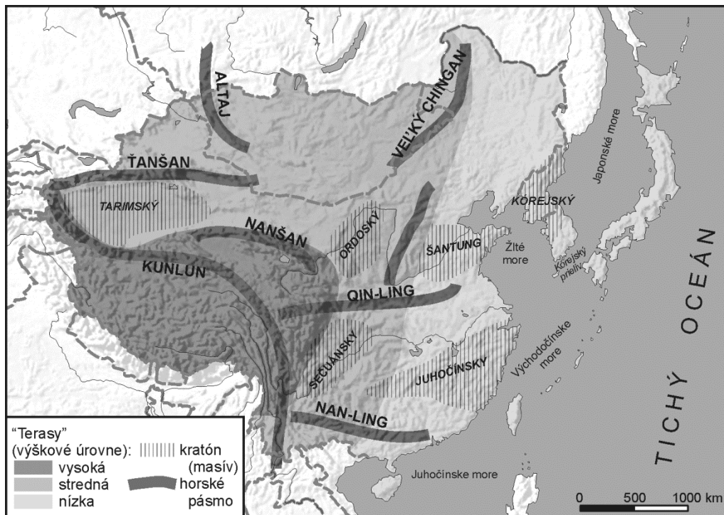
Obr. 51 Základná tektonická stavba východnej Ázie
