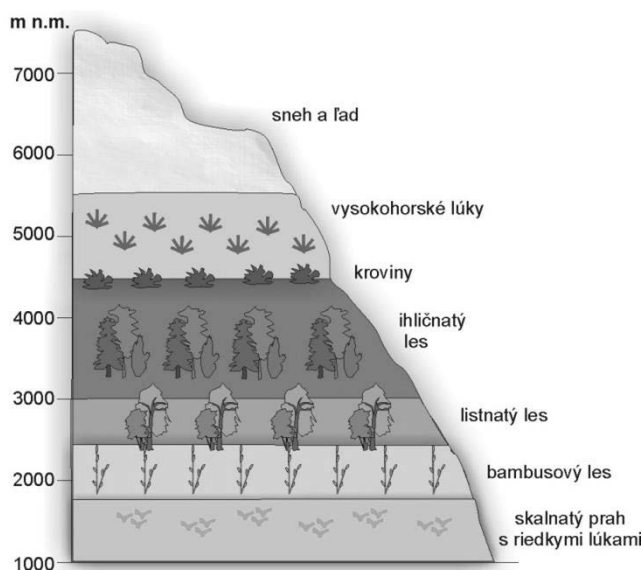
Obr. 54 Výškové vegetačné stupne na Gongga Shan
